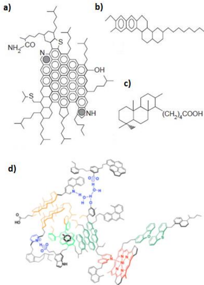
Figure 2 Exemples de structures moléculaires : a) asphaltène à structure condensée, b) résine, c) acide naphténiq, et d) asphaltène à structure dispersée (Langevin et collab., 2004 ; University of Alberta, s.d.)
